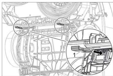
1 Goupille de retenue
