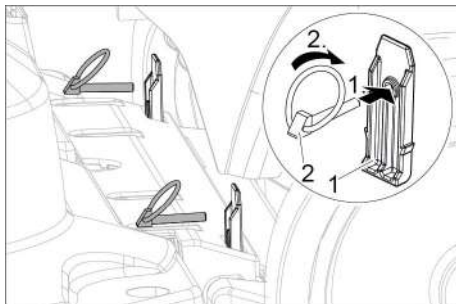
1 Goupille de retenue 2 Goupille
